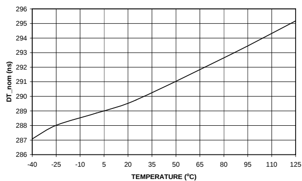
Figure 12. T_dead_nom
