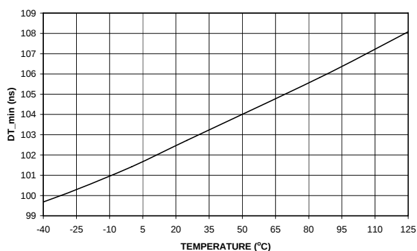
Figure 11. T_dead_min
