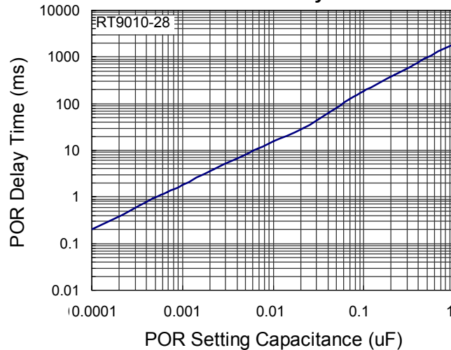
POR Delay
