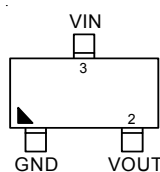
SOT-23-3
