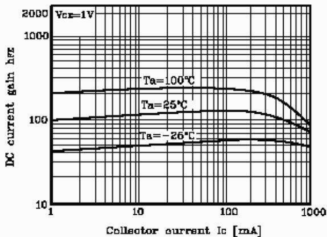
Fig. 5 h_{FE} - I_C
