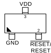
SOT-23-3
